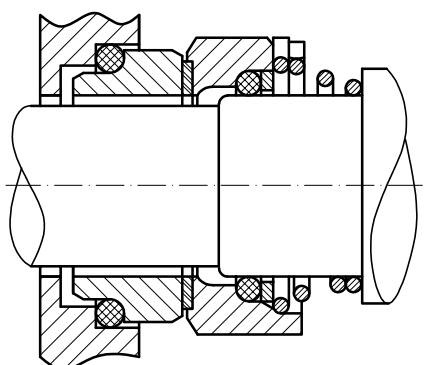
BT-1.3 Karbid volframa, ulemeljen u rotirajući prsten
