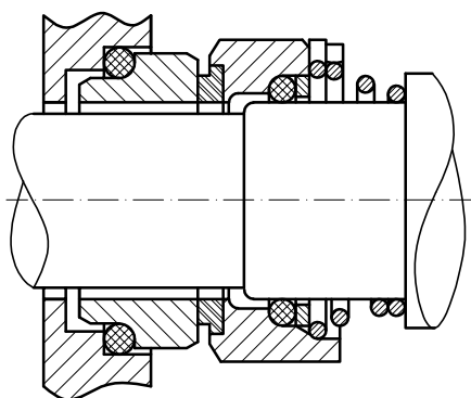
BT-1.1 Karbon grafit, utisnut u rotirajući prsten
