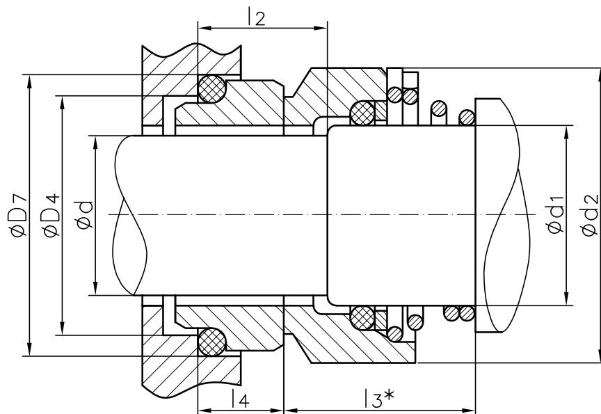
BT-1.1 Karbon grafit, utisnut u rotirajući prsten
