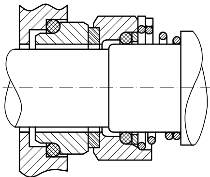
BT-1.2 karbid silicijuma, utisnut u rotirajući prsten
